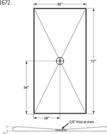
36" x 72" HBLPSP3672
