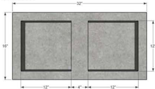
32" x 16" HBRDWSN3216
