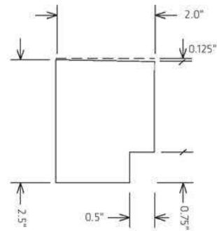
60" HBSCM60 / 84" HBSCM84
