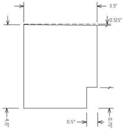
60" HBSC60 / 84" HBSC84
